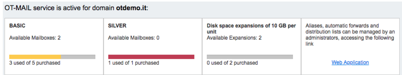
Figura 3: Resoconto risorse
